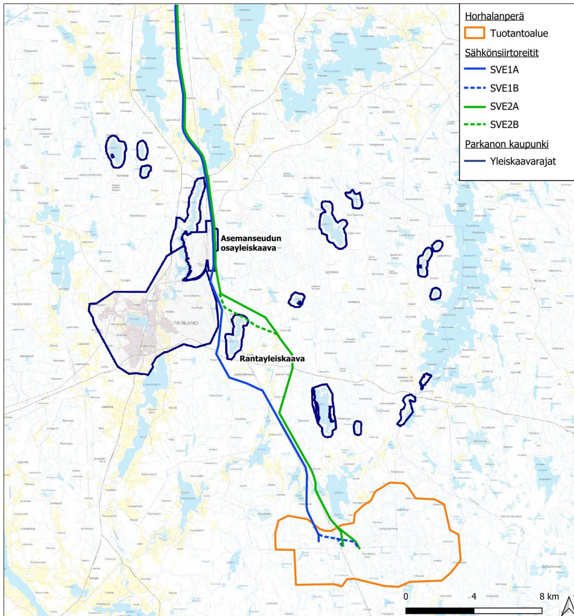
Kuva 8: Tuotantoalueen (kaava-alueen) rajausta sekä sähkösiirtoreittien sijoittuminen Parkanon kaupungin yleiskaava-alueelle.
