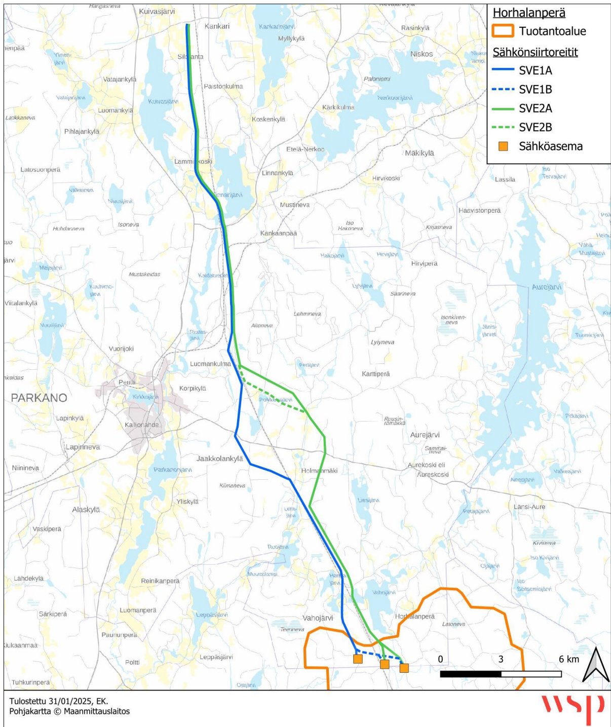
Kuva 3: Alustavat sähkönsiirtoreitit ja sähköasemat on esitetty yllä olevassa kuvassa. Sähkönsiirtoreitit ja tuotantoalueen rajat ovat alustavia ja voivat vielä muuttua YVA-menettelyn aikana tehtävien selvitysten tulosten perusteella.
