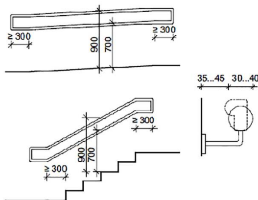
Käsijohteen mitoitus RT 103027 Portaat ja luiskat
