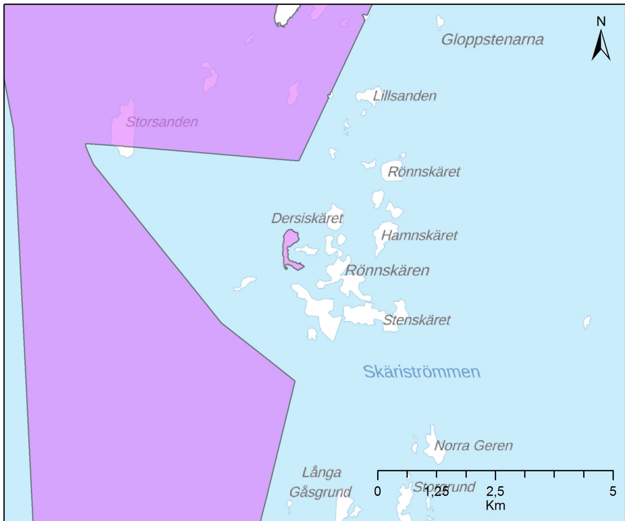
Karta 5. Beredningsområdet för naturskyddsområdet i Kvarken: Malax, Rönnskären. Kartta 5. Valmisteltava luonnonsuojelualue Merenkurkussa: Malax, Rönnskären.
