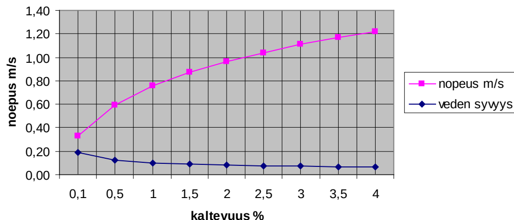
Kaltevuuden muutoksen vaikutus virtausnopeuteen
