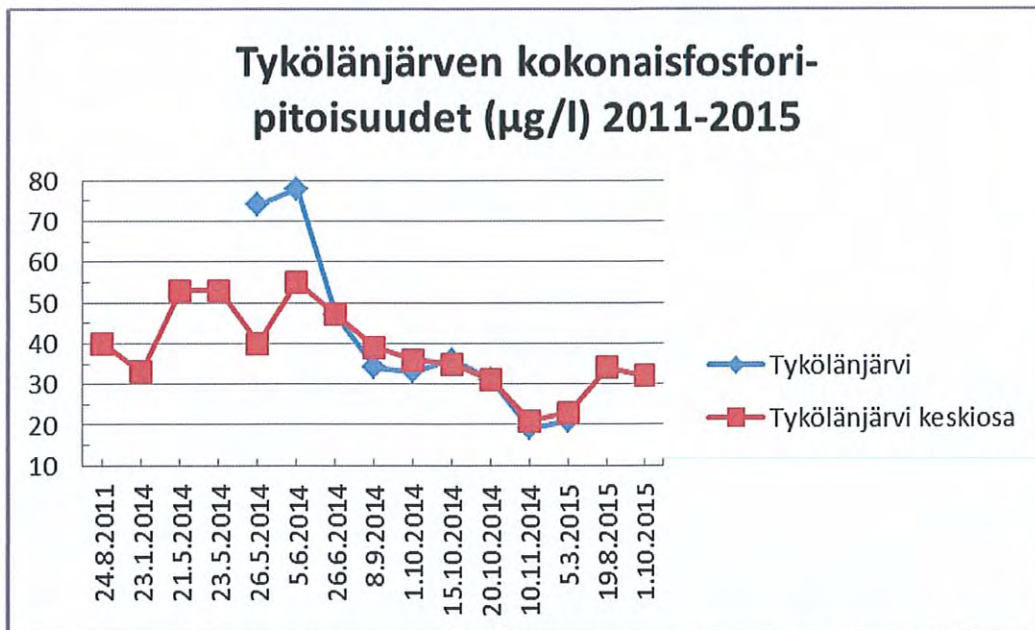
Kuva 4. Kokonaisfosforipitoisuudet Tyköljänjärnessä (Tyköljänjärvi ja Tyköljänjärvi keskiosa) vuosina 2011-2015.
