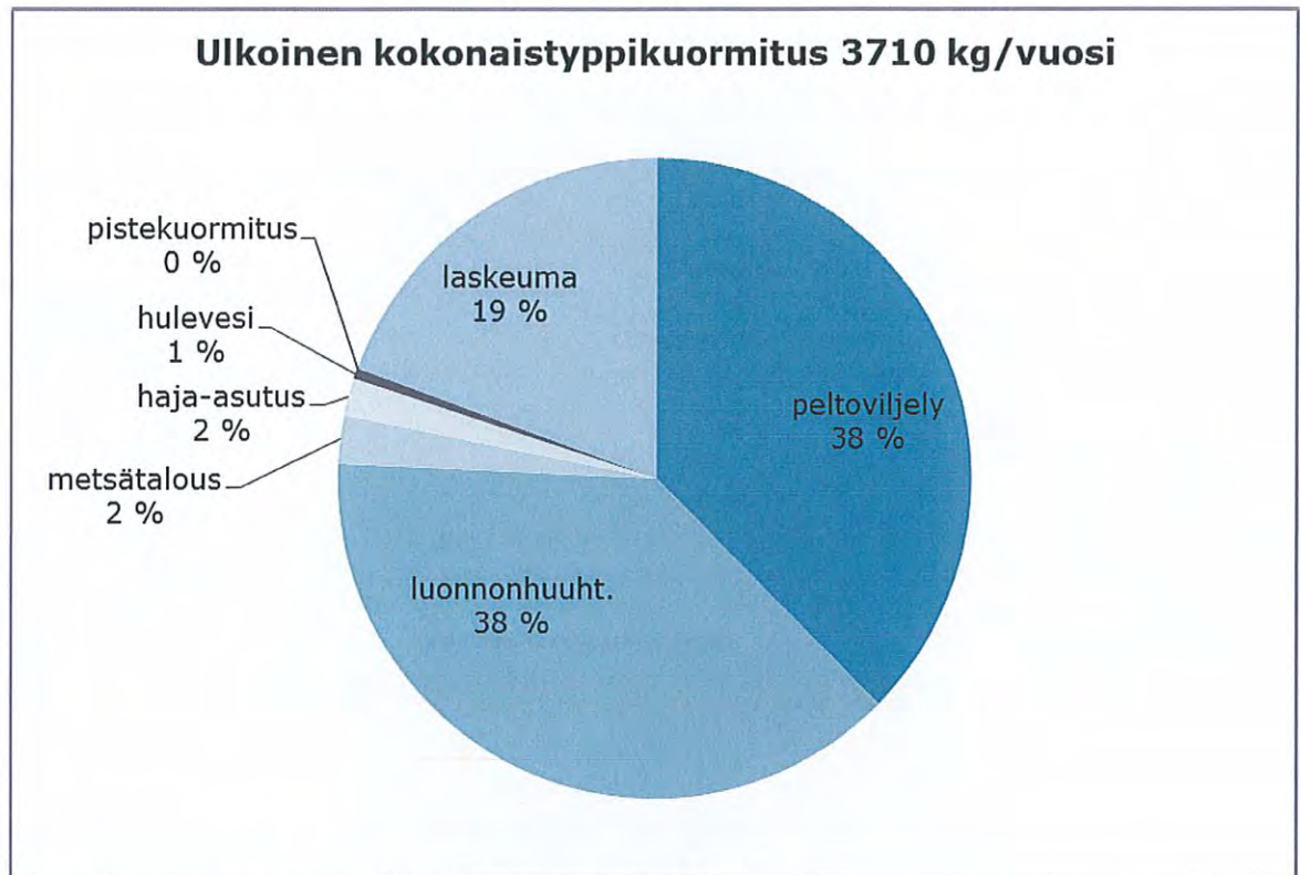
Kuva 13. Tyköljänjärven kokonaistyyppikuormitus.
