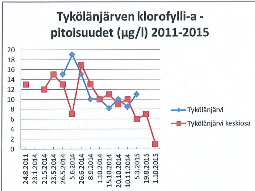
Kuva 6. Klorofylli-a -pitoisuudet Tyköljänjärvessä (Tyköljänjärvi ja Tyköljänjärvi keskiosa) vuosina 2011-2015.
