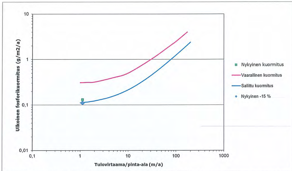
Kuva 14. Vollenweiderin kuormituksen sietorajat, Tyköljänjärven nykyinen kuormitus.
