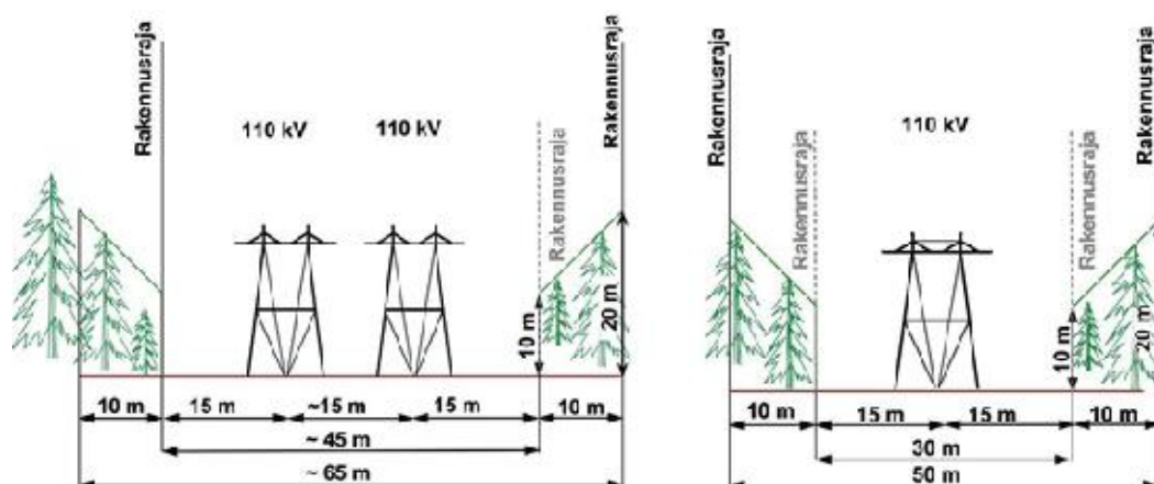
Kuva 3. Yhden tai kahden rinnakkain rakennetun 110 kV:n voimajohdon tyyppiinirustus
