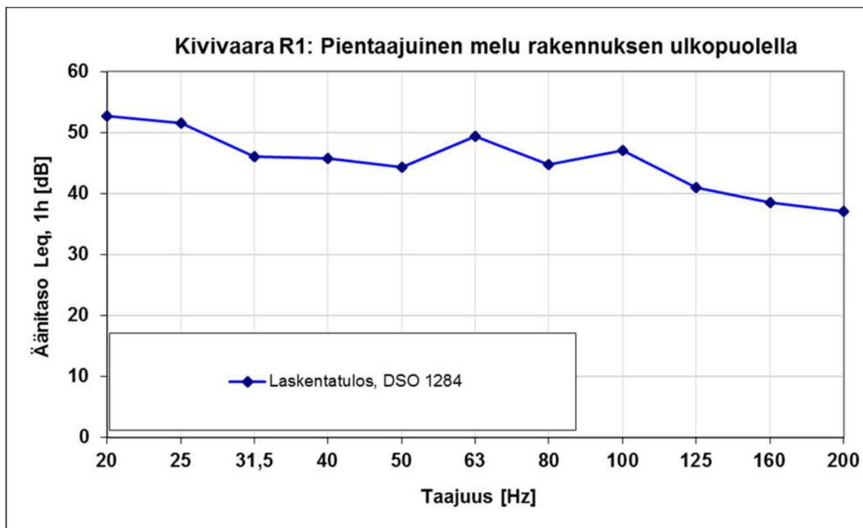
Kuva 31. Pientaajuinen melu rakennuksen ulkopuolella meluselvityksen kohteessa R1 (Suomussalmi, eräkämpä).
