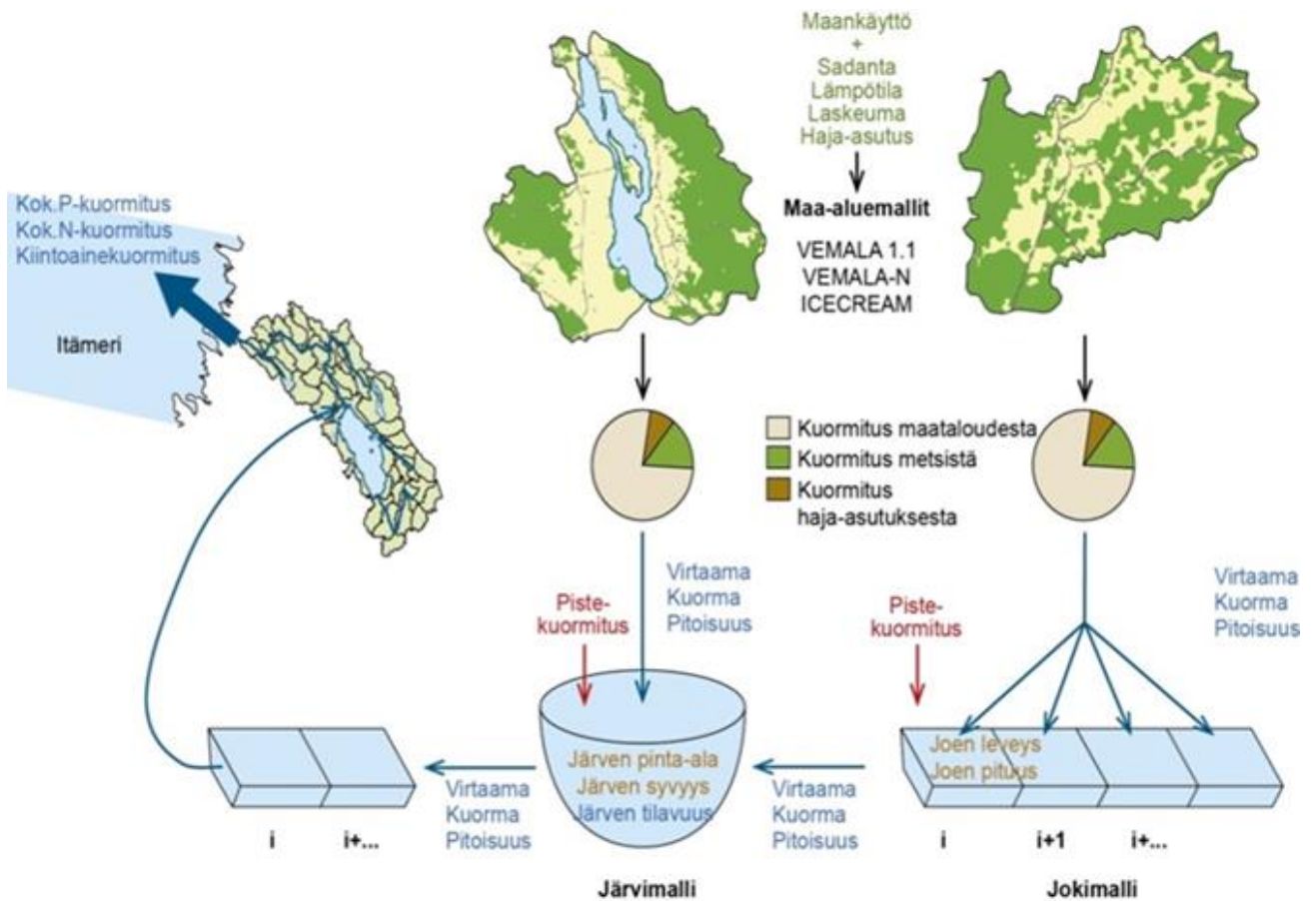
Kuva 1. NIM malliperhe.
