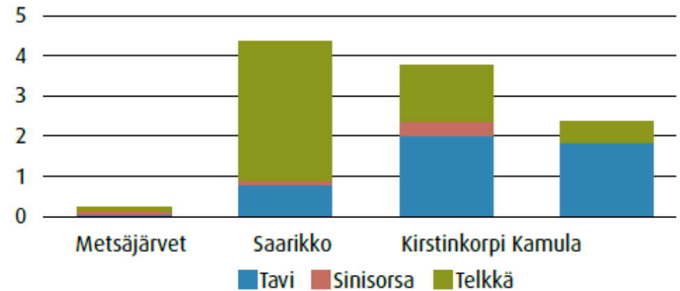
Poikuetiheys REAH-kosteikoilla ja muilla kosteikoilla
