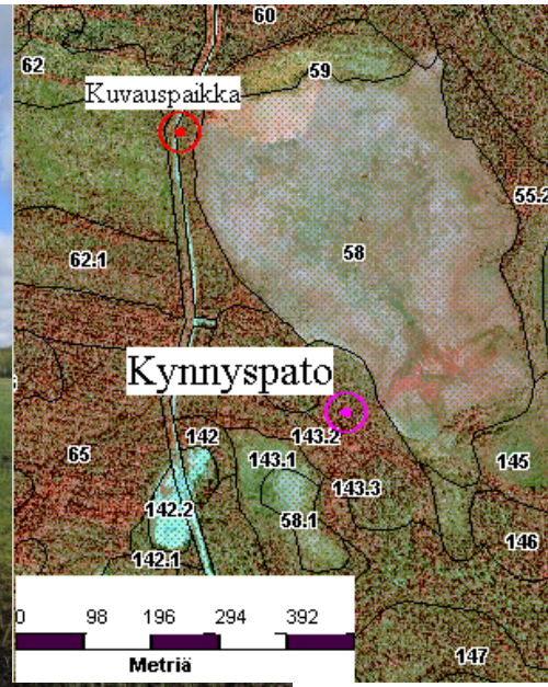
Kinttaislampi Pudasjärvi v.2010 Kuivattu 1910 – 1920 luvulla
