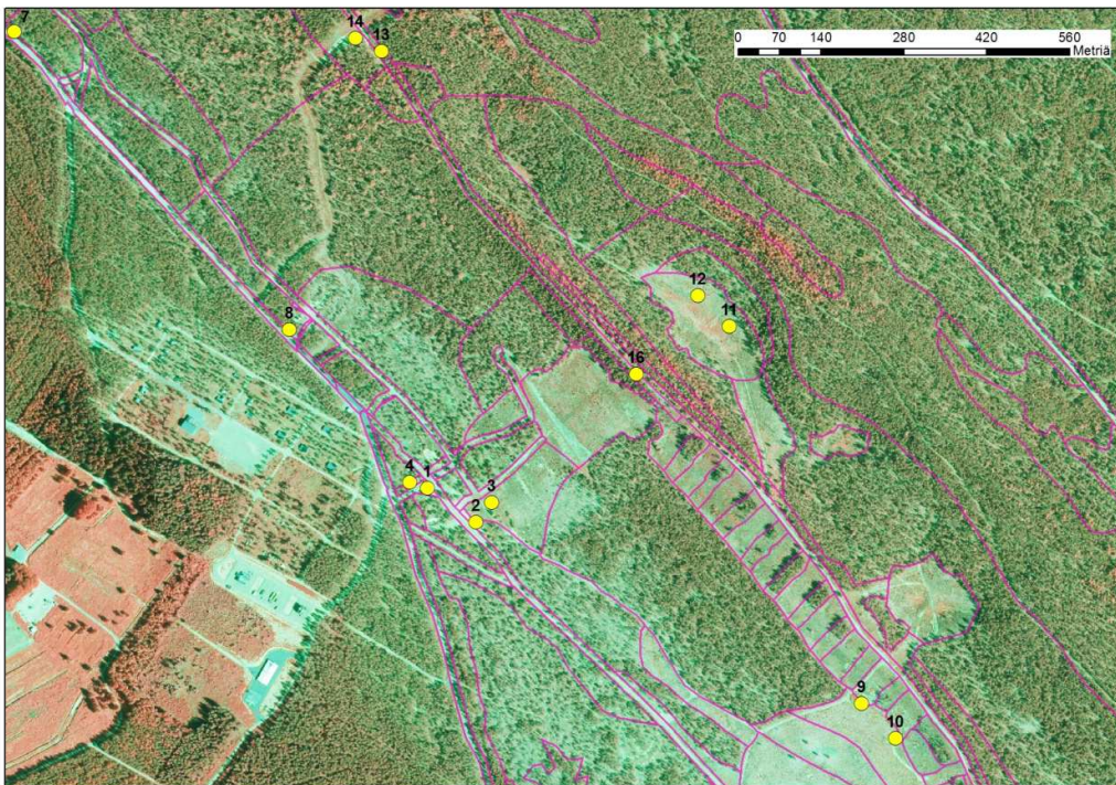
Kartta 2. Hankkeen hoitoalueella olevat esiintymät.
